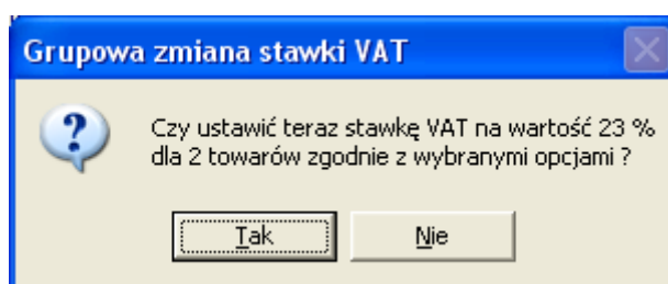
Rys 3.10 Pytanie potwierdzające
