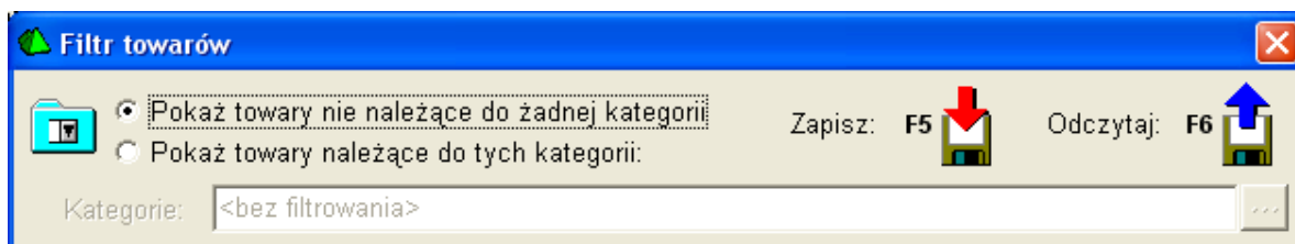
Rys 3.4 Filtr towarów
